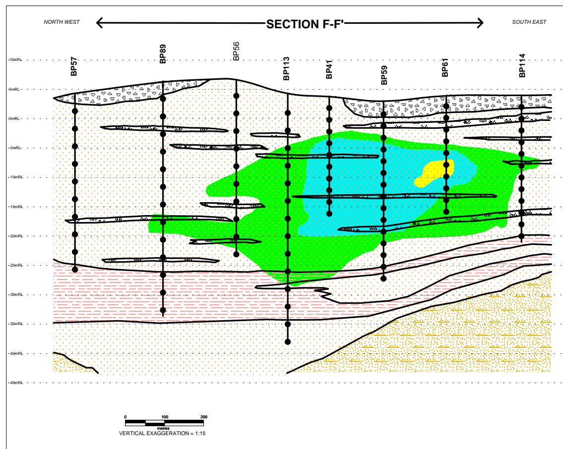
CHLOROFORM
